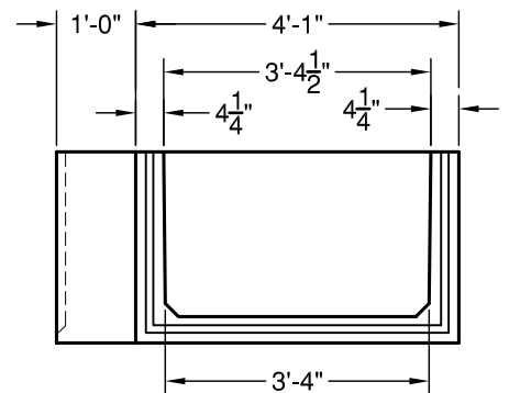
ELEVATION BB
