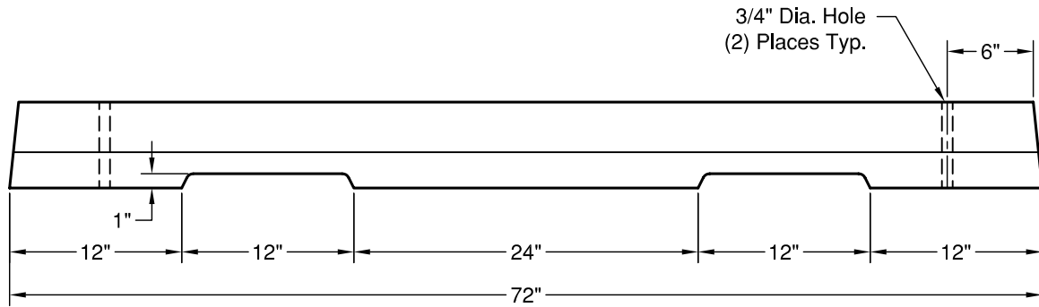
ELEVATION
